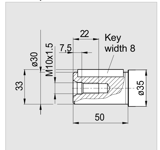
Parallel Keyed Shaft: DIN 6885 8x7x40
